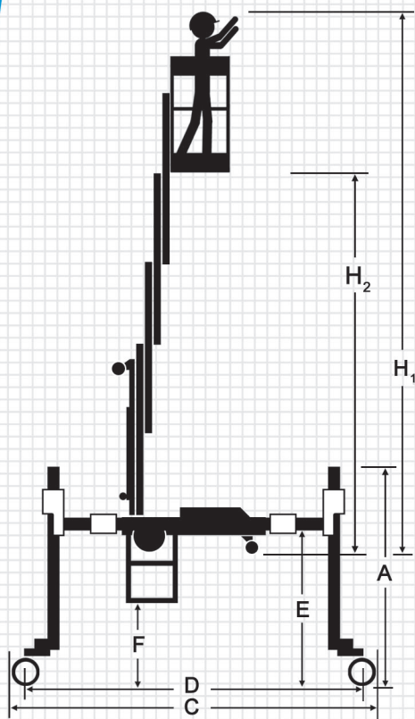
نمای جانبی دستگاہ با پایہ مخصوص در حالت باز شدہ Side Plan with special base in Unfolded Status
