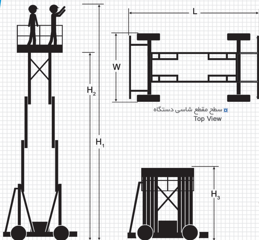
نمای جانبی دستگاه در حالت باز شده Side View in Unfolded Status
